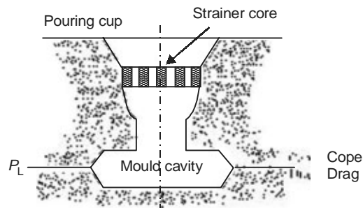
Fig. 5.11: Top Gate
