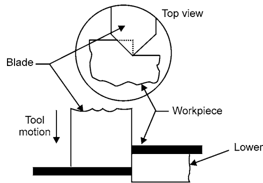
Fig. 4.33: Notching
